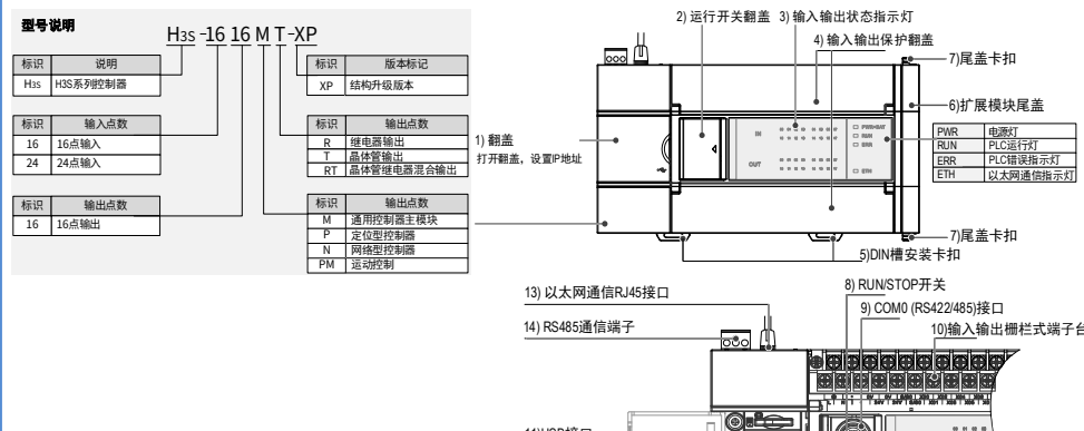
图2 H 3S -1616MT-XP/H 3S -2416MT-XP 产品外观及型号说明
